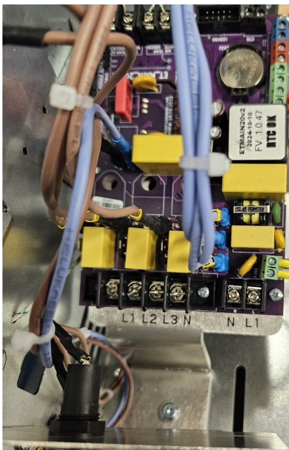
Rys. 10. Płyta sterownika zamontowana w komorze sterującej ogrzewacza
