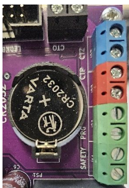
Rys.12. Zdjęcie zacisków CTZ/P oraz CTP/P
